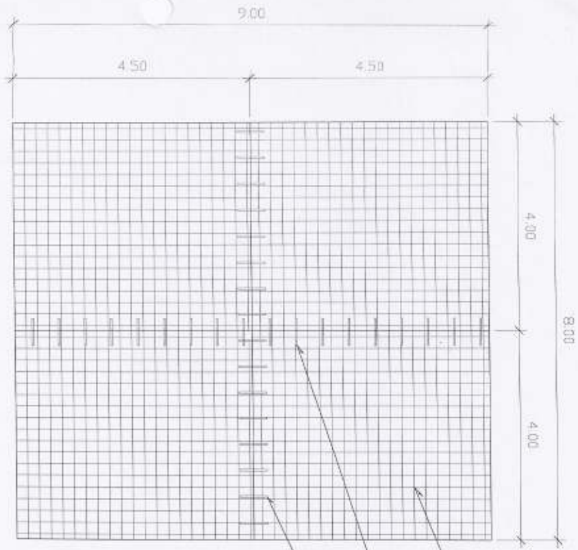
แบบแสดงการเสริมเหล็ก
